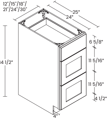
12", 15", 18", 21", 24", 30" 3 DRAWERS
