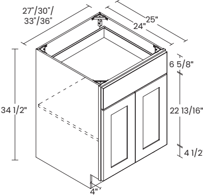
27", 30", 33", 36" 2 DOORS / 1 DRAWER
