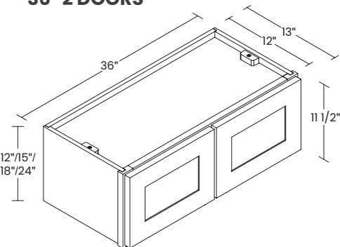
36" 2 DOORS
