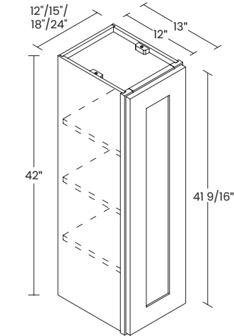
42" HIGH 1 DOOR
