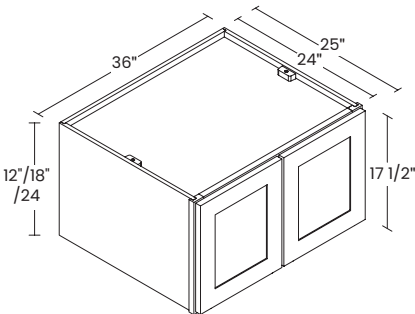
36" 2 DOORS
