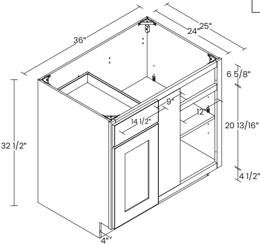
36" BASE BLIND CORNER 1 DOOR / 1 DRAWER
