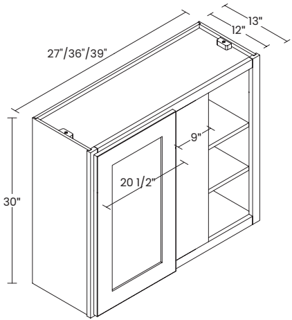
30" HIGH 1 DOOR
