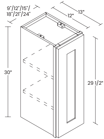
30" HIGH 1 DOOR
