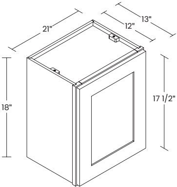
21" 1 DOOR
