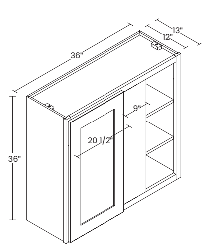
36" HIGH 1 DOOR
