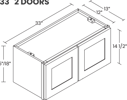
33" 2 DOORS
