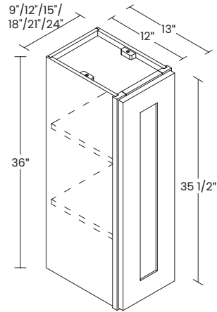
36" HIGH 1 DOOR
