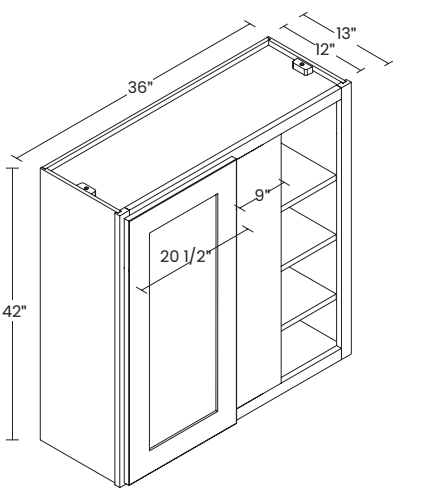
42" HIGH 1 DOOR
